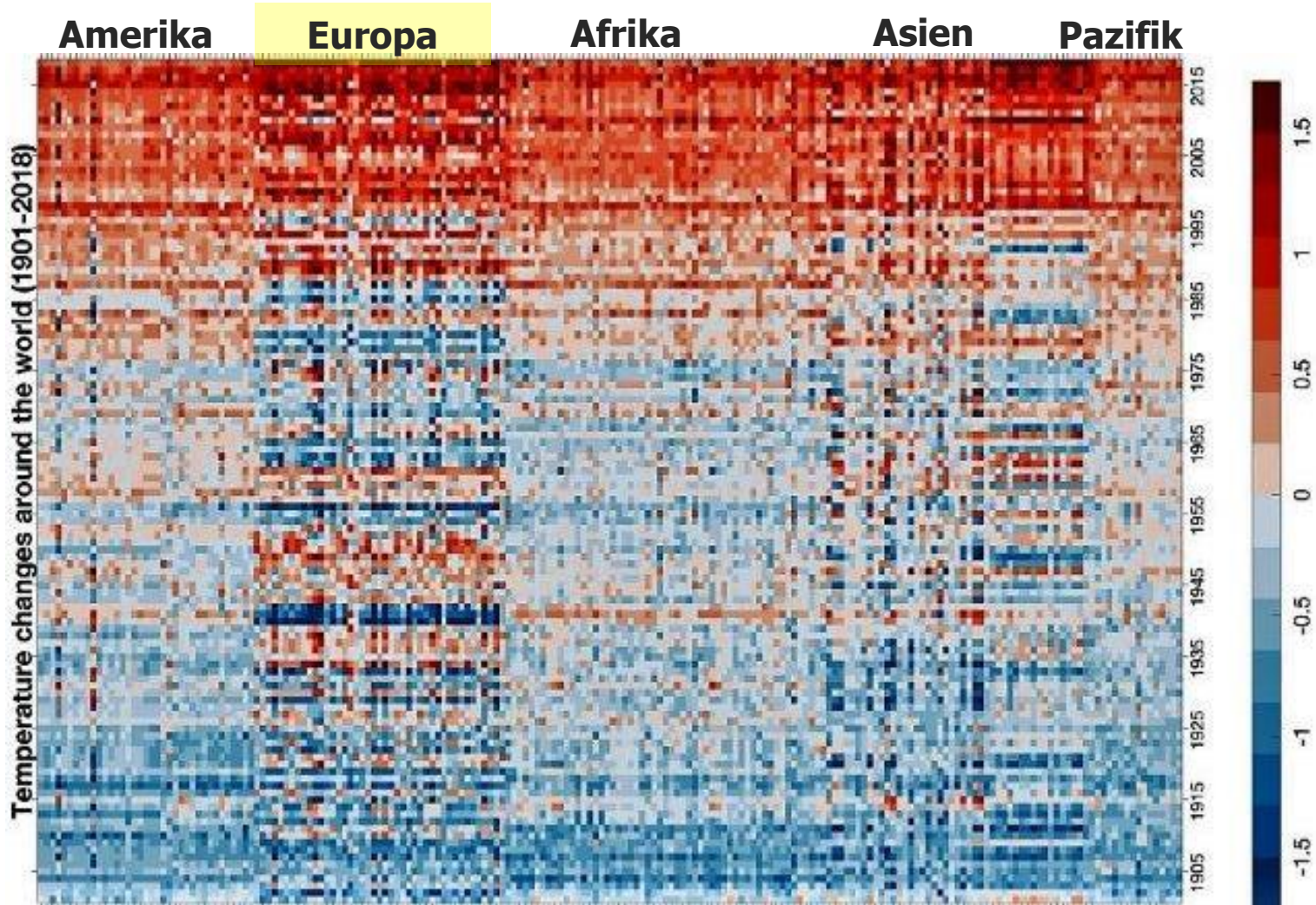
Visualisierung der Jahresdurchschnittstemperaturen in Streifenmustern (Klimaforscher Ed Hawkins, University of Reading)
